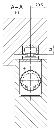
Querschnitt
