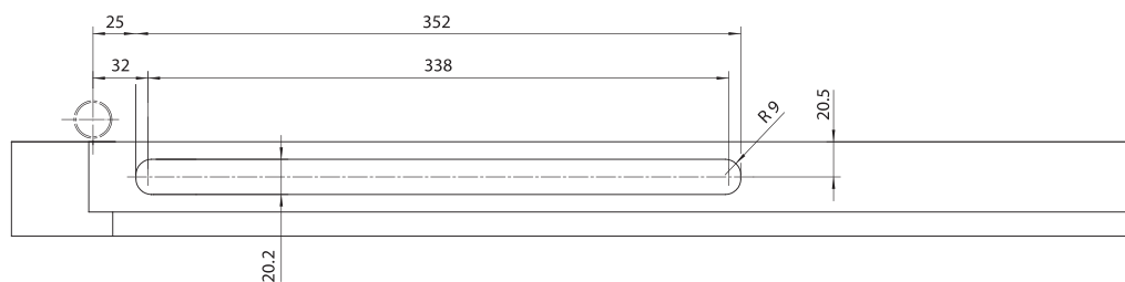
Bearbeitung Türzarge
