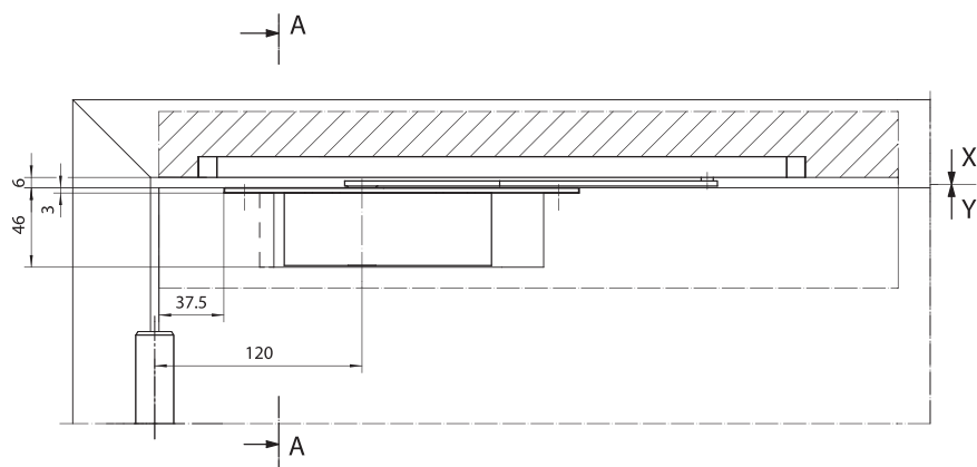
Längsschnitt
