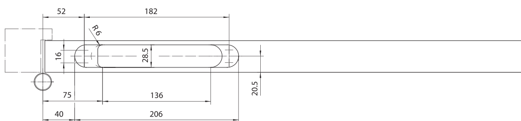
Bearbeitung Türblatt
