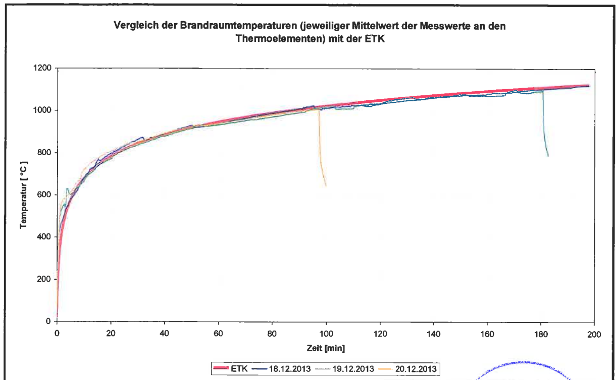
Bild 1: Brandraumtemperaturen
