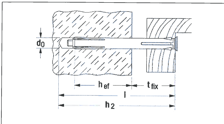
Bild 2: Einbauskeizze nach [2]
