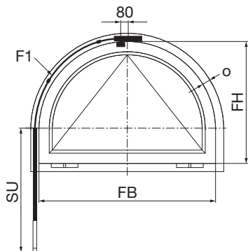
Rundbogen, 1 Schere
