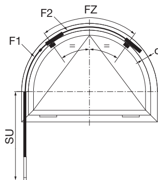
Rundbogen, 2 Scheren
