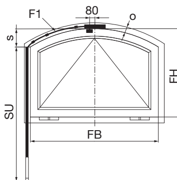
Flachbogen, 1 Schere
