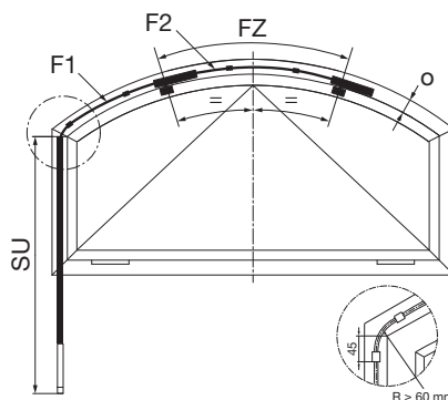
Flachbogen, 2 Scheren
