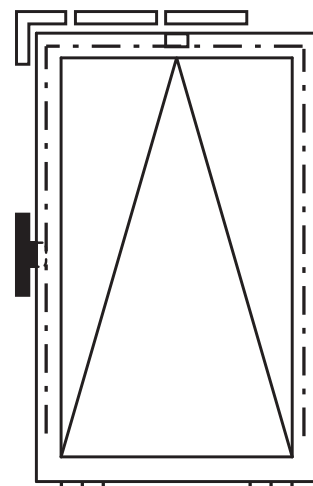
Seitliche Kupplung ZV/F FB: 440 - 620 mm FH: mind. 500 mm
