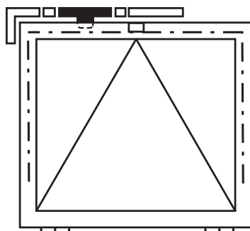
Oben liegende Kupplung ZV/F FB: 621 - 2400 mm FH: mind. 300 mm
