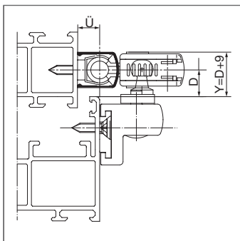
GEZE OL 95 an Leichtmetallfenster mit Überschlag
