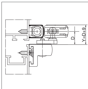
GEZE OL 95 an Leichtmetallfenster glattschlagend
