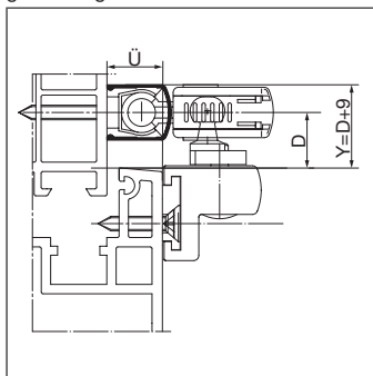
GEZE OL 95 an Kunststofffenster
