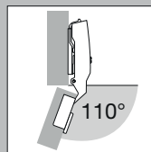
Sensys 8645i / 8675 (effektiver Öffnungswinkel = 100°)
