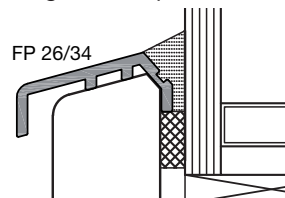
Flügelabdeckprofil FP 26/34
