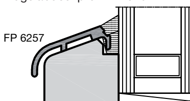
Flügelabdeckprofil FP 6257
