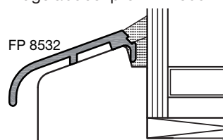
Flügelabdeckprofil FP 8532
