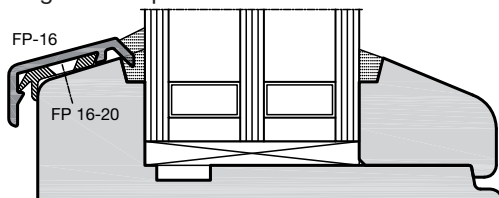
Flügelabdeckprofil FP 16
