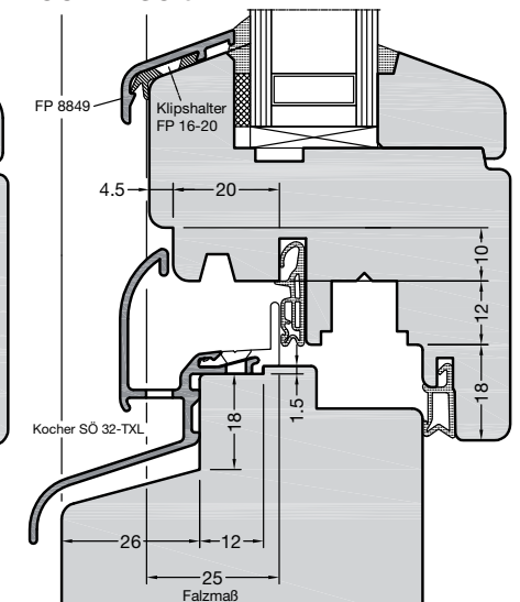
KOCHER SÖ 32-TXL
