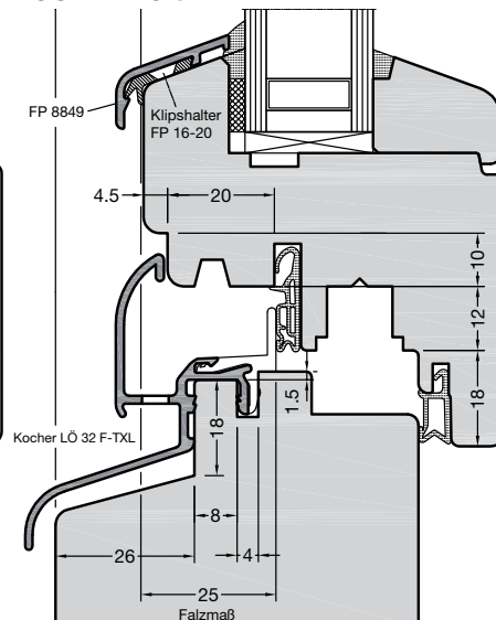
KOCHER LÖ 32 F-TXL
