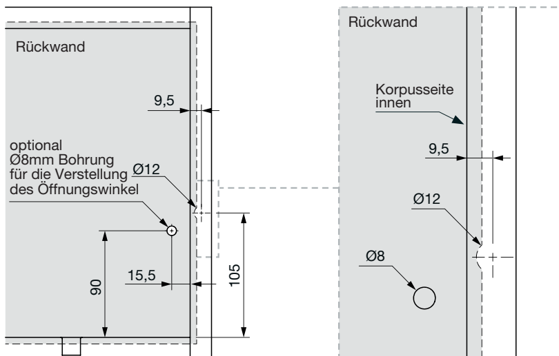
Bohrplan Rückwand
