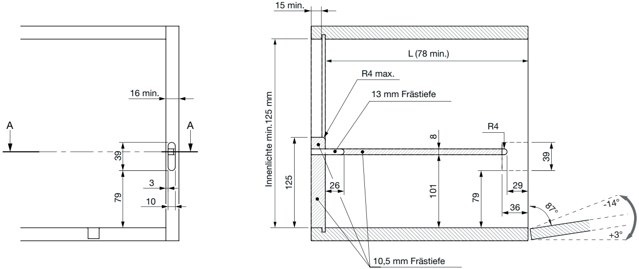
Bohrplan Korpusseite
