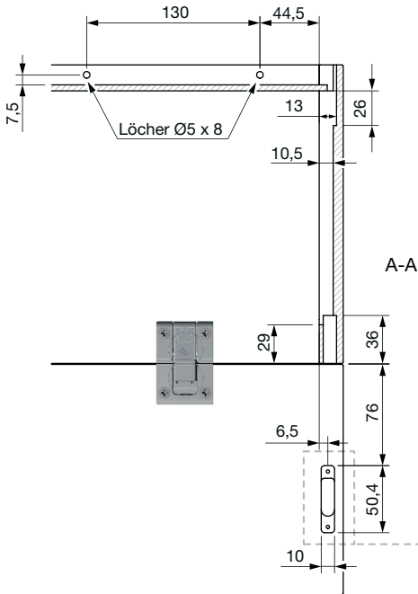
Bohrplan Rückwand
