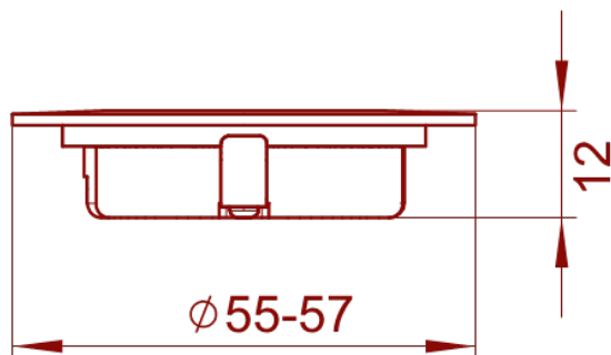
Rysunek techniczny
