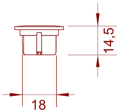
Tehnična risba
