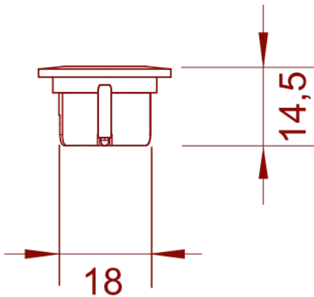
Technische Zeichnung
