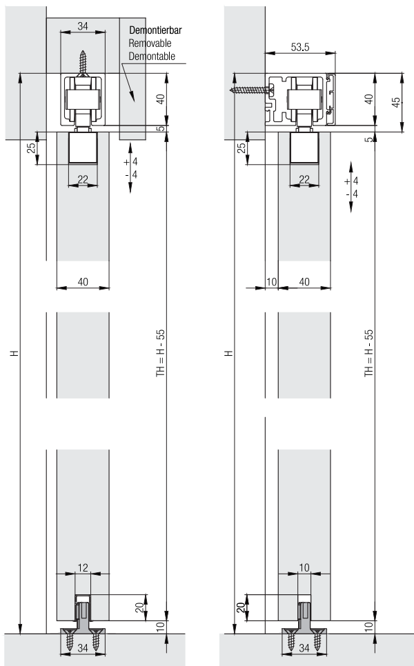
Einzugsdämpfung SoftMove 100
