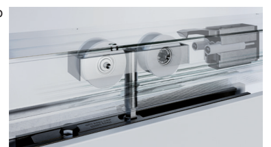
Rollapparat mit SoftStop
