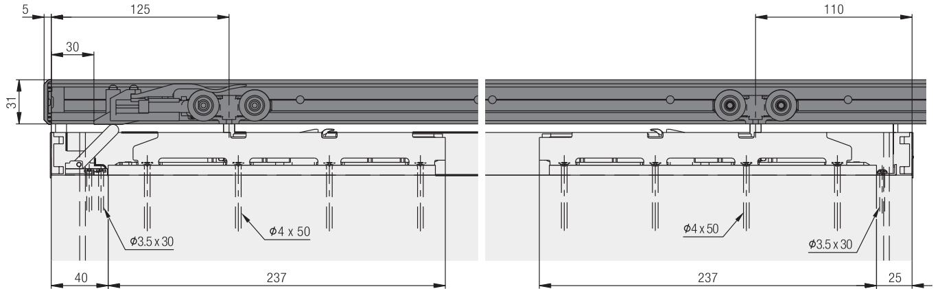
Ansicht teilöffnend
