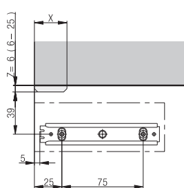
Montagedetail Bodenführung
