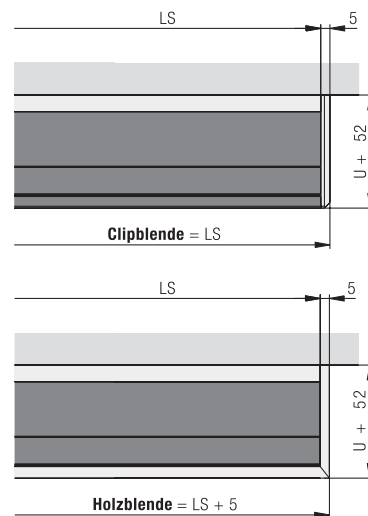
Berechnung Clipblende / Holzblende
