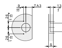
DETAIL F 2:1
