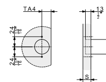
DETAIL E 2:1
