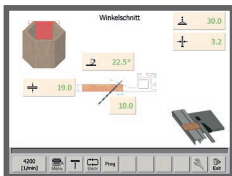
Winkelschnitt
