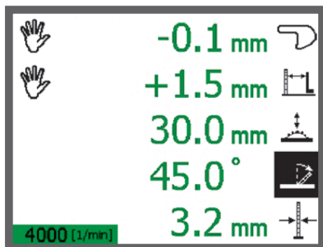
Maschine in Grundausstattung, geschwenktes Sägeblatt, manuelle Maßkorrektur
