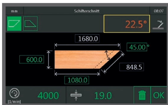
Schifterschnitt
