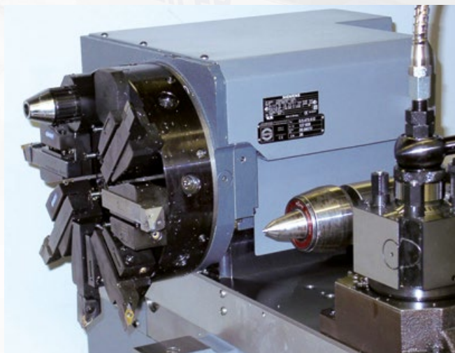
8-fach-Scheibenrevolver ohne/mit Werkzeugantrieb
