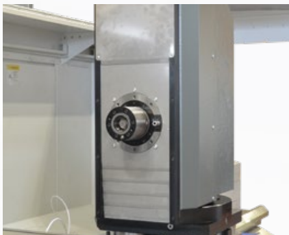
Y-Achse 200 mm Hub (nur bei E110/E120)
