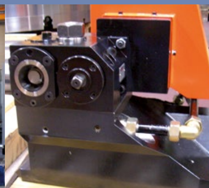
Werkzeugträgerkopf mit angetriebenen Werkzeugen, Aufnahme Capto C8
