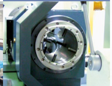
Ringlünette mit 270 mm Durchmesser
