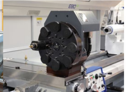
8-fach-Scheibenrevolver mit angetriebenen Werkzeugen, Schaft- \varnothing 40 mm
