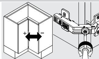
Einstellung Fuge +7.2 mm -4.2 mm
