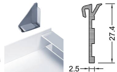
Dichtstück und Anschlussdichtung UD 40-25
