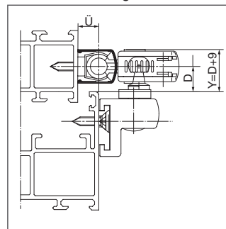
GEZE OL 90 N an Leichtmetallfenster mit Überschlagn
