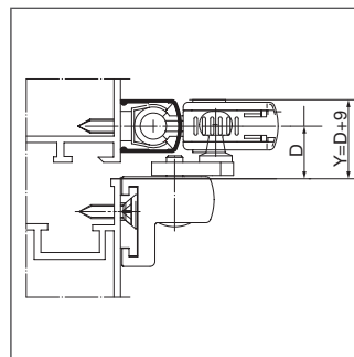
GEZE OL 90 N an Leichtmetallfenster glattschlagend
