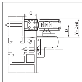
GEZE OL 90 N an Kunststofffenster
