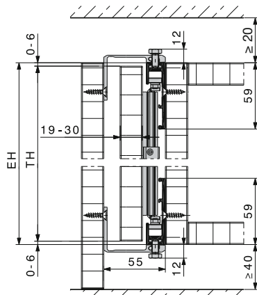
System: HAWA-Concepta 25/30 Verbindung: Connector 55 mm
